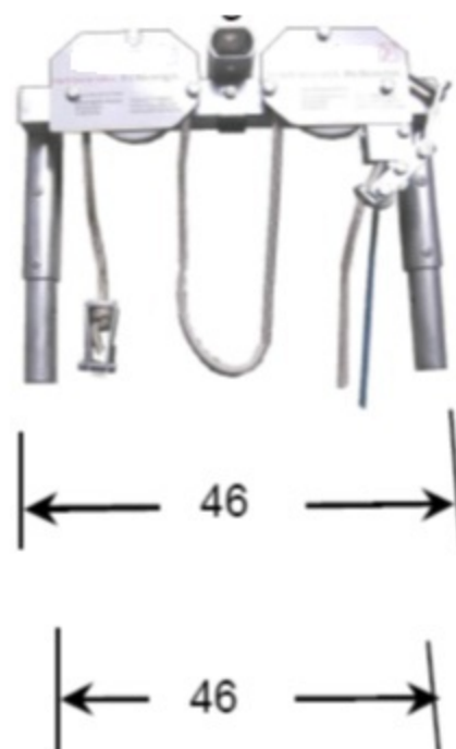
Механический привод тележки 60кг
