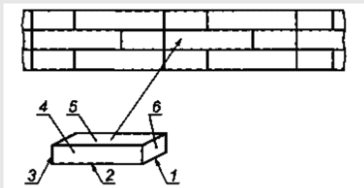
1 — ширина; 2 — длина; 3 — толщина; 4 — ложок; 5 — постель; 6 — тычок
