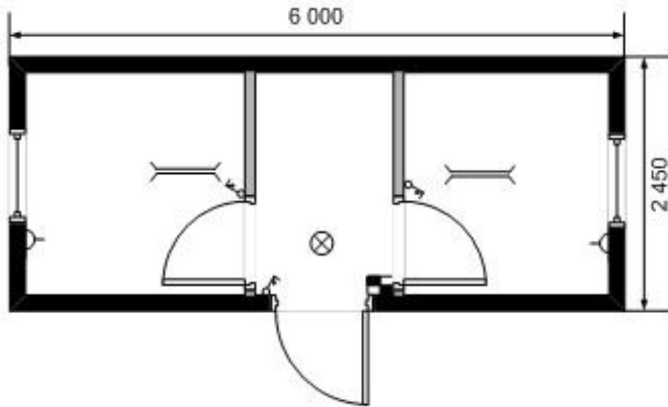
Спецификация Блок-контейнера БК-1
