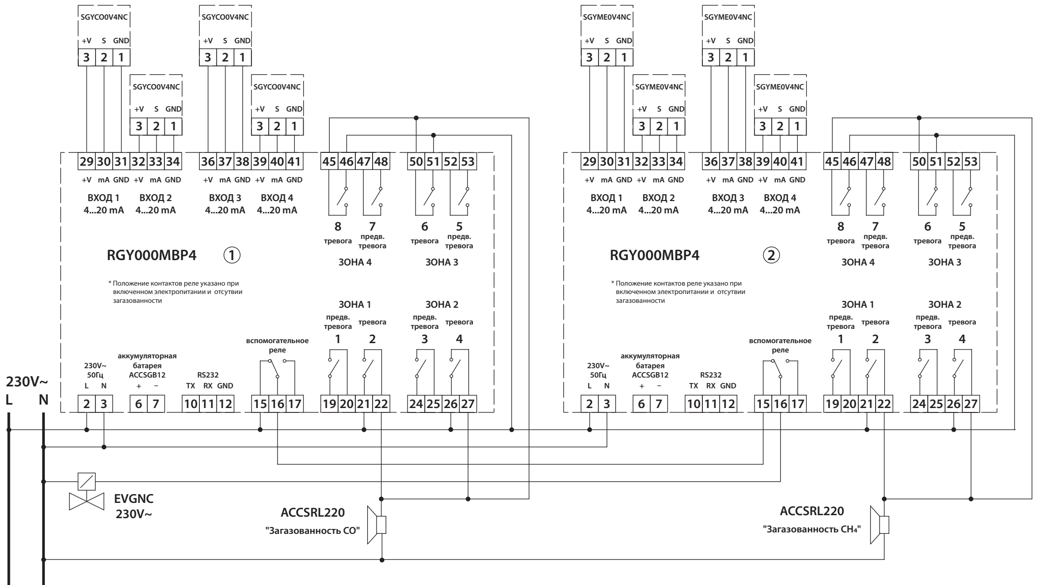
Схема соединения сигнализаторов RGY000MBP4 с внешними сенсорами SGY, с нормально-закрытым клапаном EVGNC и электронными сиренами ACCSRL220
