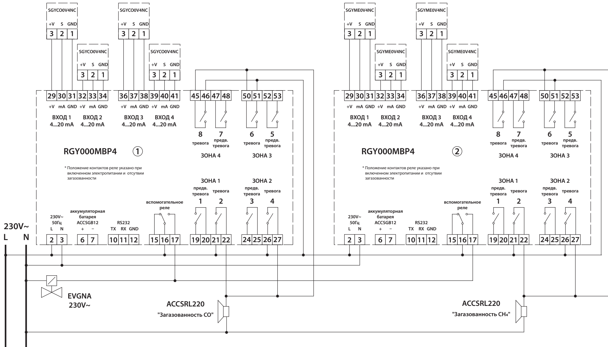
Схема соединения сигнализаторов RGY000MBP4 с внешними сенсорами SGY, с нормально-открытым клапаном EVGNA и электронными сиренами ACCSRL220
