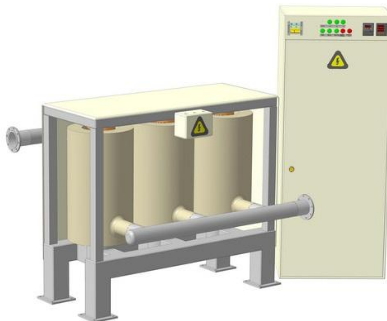
Рисунок 2 – Индукционный котел “ИКН” (внутренний вид)
