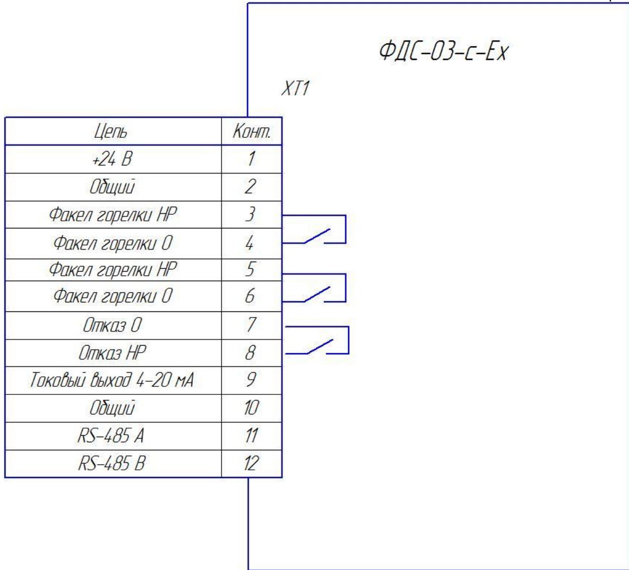
Рис.4 Схема подключения внешних цепей ФДС-03-с-Ех.
