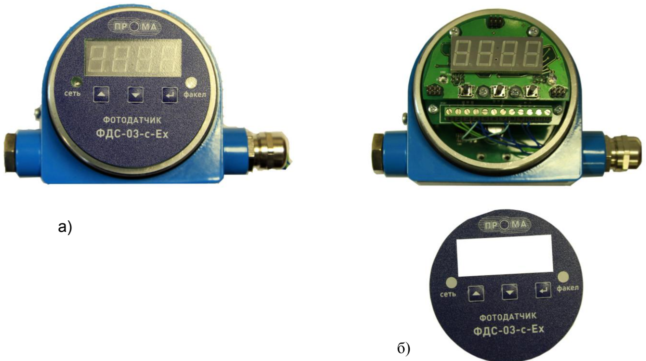
Рис. 6 Фотодатчик ФДС-03-с-Ех со снятой верхней крышкой, установленной (а) и снятой (б) передней панелью.
