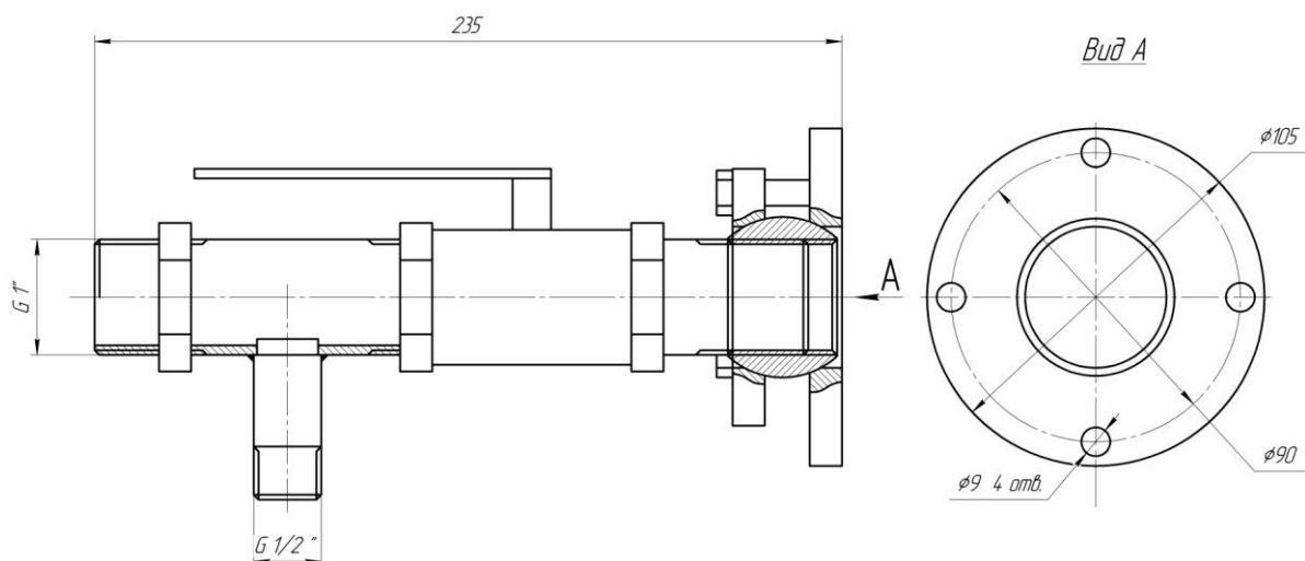
Рис.5б. Фланец монтажный юстировочный для ФДС-03-с-Ех.
