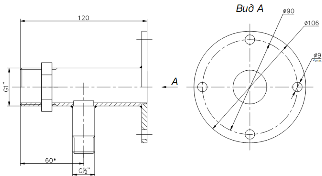
Рис.5а. Фланец монтажный для ФДС-03-с-Ех.
