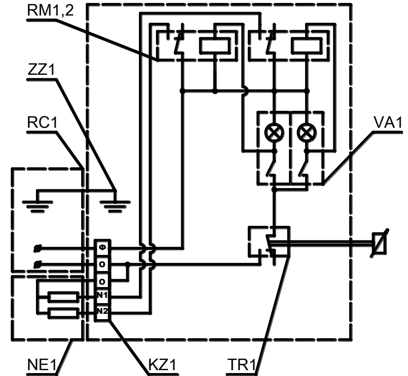
Рисунок 2 Схема ПУЭ-6
