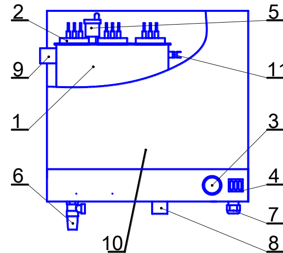
Рисунок 1. Схема электрокотла.
