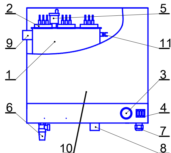
Рисунок 1. Схема электрокотла.
