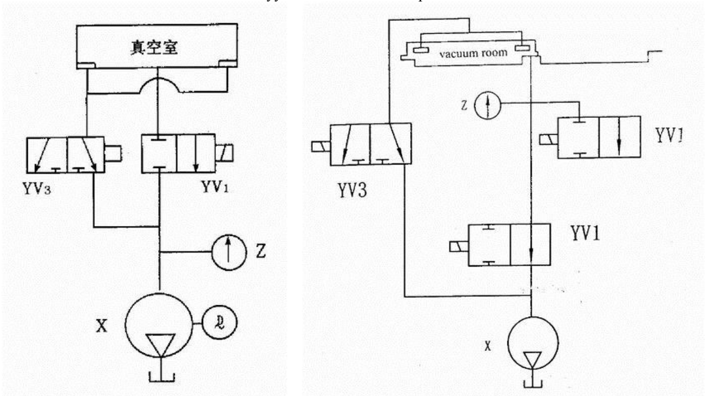
Однокамерный вакуумный запайщик с аэрацией
