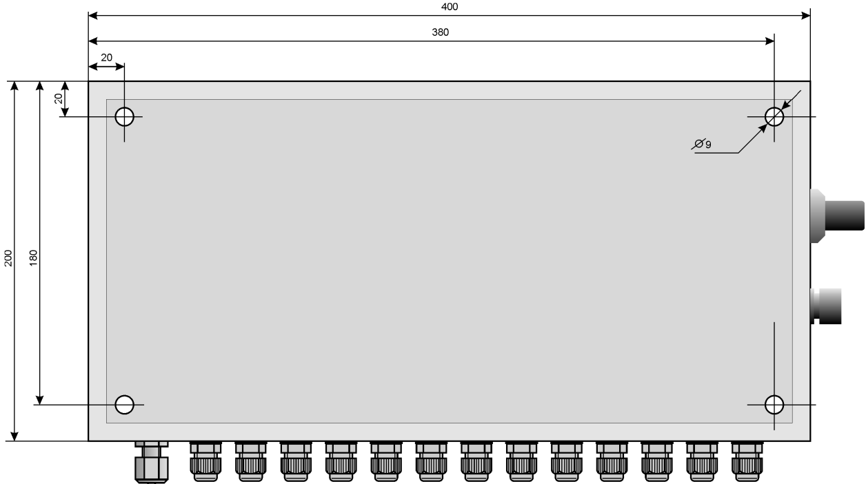
Рис. 3. Установочные размеры контроллера.
