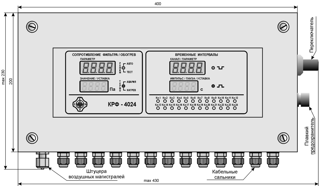
Рис.2. Габаритные размеры контроллера.
