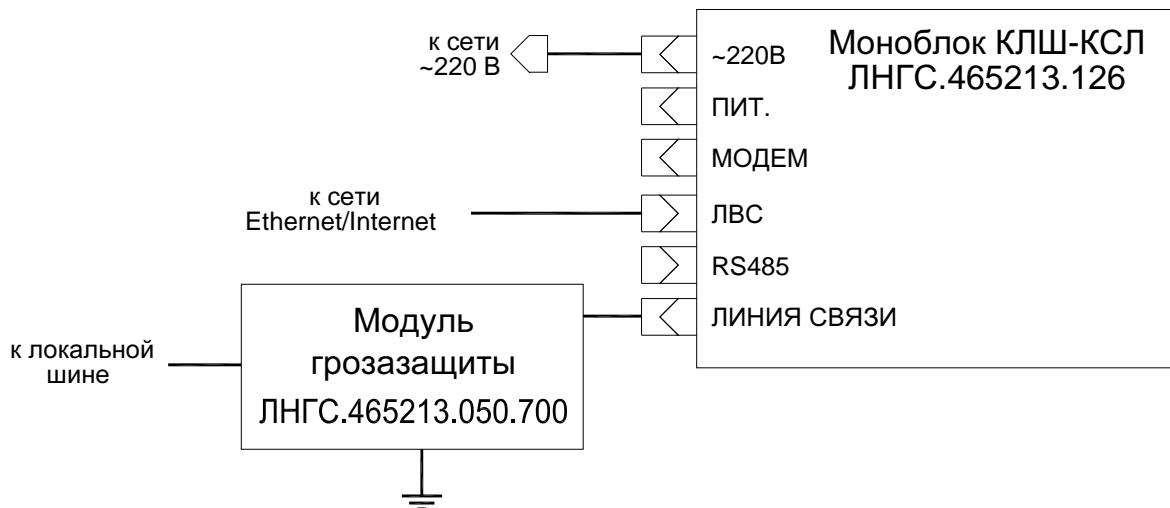
Рисунок 1. Схема подключения моноблока КЛШ-КСЛ СМ3 Ethernet (ЛНГС.465213.126)
