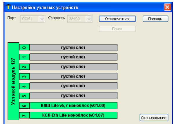
Рисунок 4. Диалоговое окно программы после подключения к моноблоку
