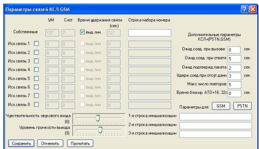
Рисунок 7. Диалоговое окно параметров связей КСЛ моноблока
