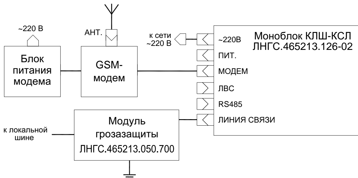
Рисунок 3. Схема подключения моноблока КЛШ-КСЛ СМ3 GSM (ЛНГС.465213.126-02)
