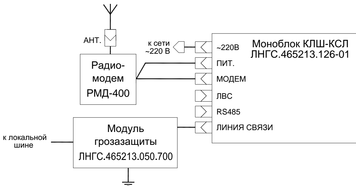
Рисунок 2. Схема подключения моноблока КЛШ-КСЛ СМ3 433 МГц (ЛНГС.465213.126-01)
