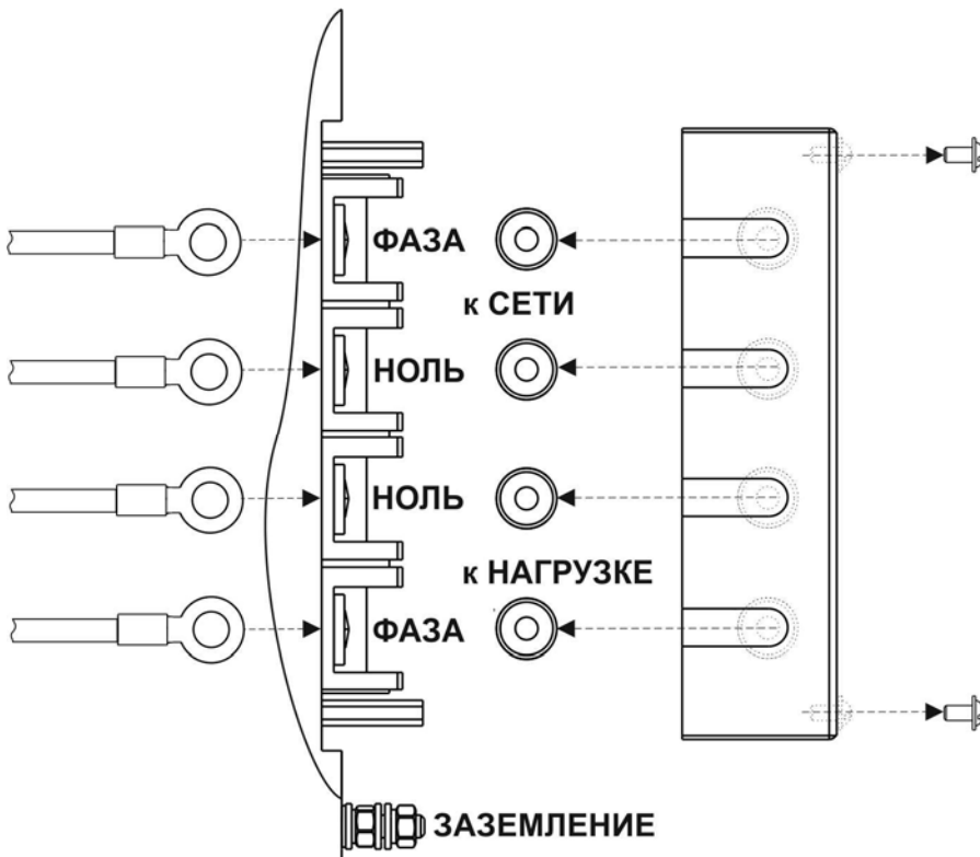
Рисунок 3. Подключение стабилизатора
