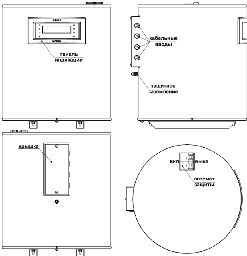
Рисунок 1. Внешний вид стабилизатора
