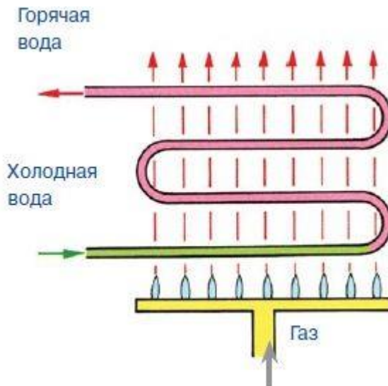
Горелка и теплообменник – основные части газового котла
