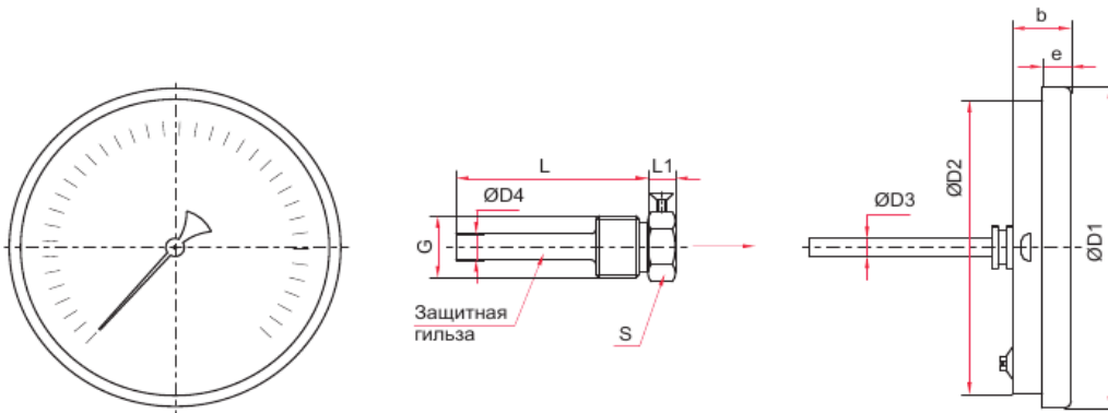
Осевое присоединение (Ø80, 100, 150 мм)
