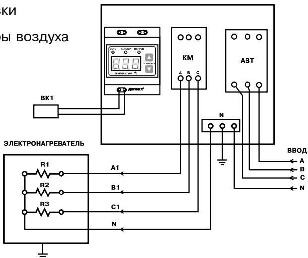
Рис.2 Схема подключения панели управления
