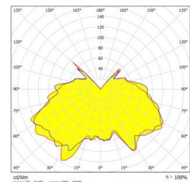
Рисунок 2 – Световое распределение лампы E27 C37 8W.
