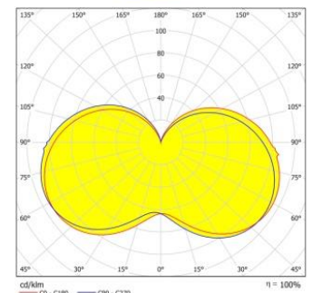
Рисунок 2 – Световое распределение лампы E14 C37 5W.
