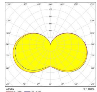
Рисунок 2 – Световое распределение лампы E14 C37 7W.
