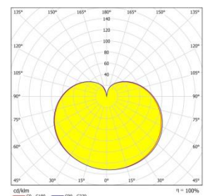
Рисунок 2 – Световое распределение лампы E27 A60 7W.
