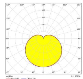
Рисунок 2 – Световое распределение лампы E27 A60 10W.
