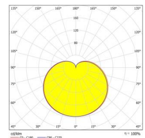
Рисунок 2 – Световое распределение лампы E27 A60 12W.
