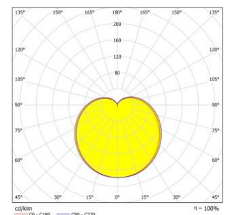
Рисунок 2 – Световое распределение лампы E14 G45 5W.
