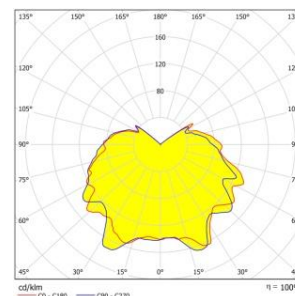
Рисунок 2 – Световое распределение лампы E14 G45 8W.
