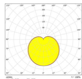
Рисунок 2 – Световое распределение лампы E27 G45 5W.
