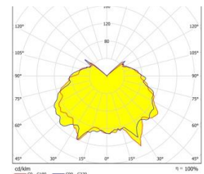
Рисунок 2 – Световое распределение лампы E27 G45 8W
