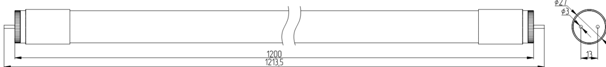
Рисунок 3 – Габаритный чертеж.
