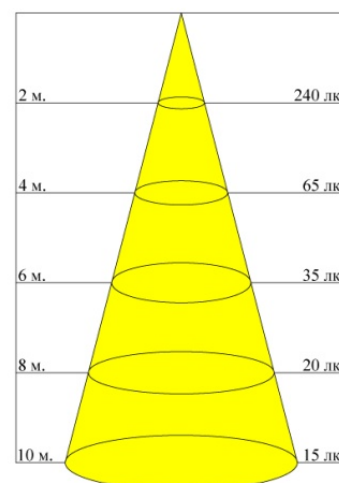
Geniled СДЛ-КС 40W (светильник с диффузор 120°)
