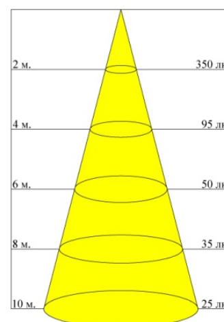
Geniled СДЛ-КС 80W (светильник с диффузор 120°)
