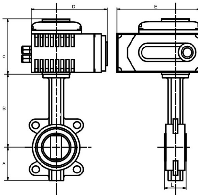
Чертеж габаритный затвора поворотного с электроприводом Сатурн, Ду40-Ду300:
