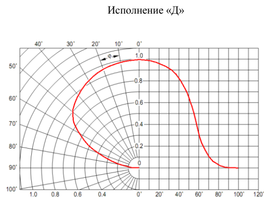
Рисунок 4 Тип КСС
