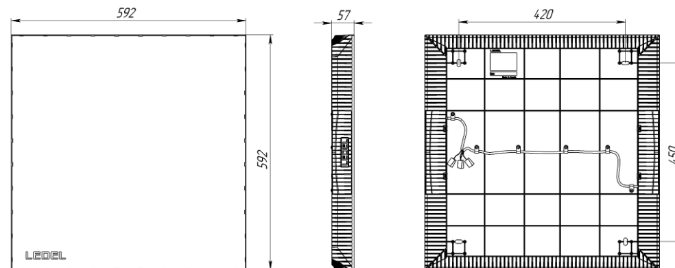
Рисунок 1 Светильник L-office 32
