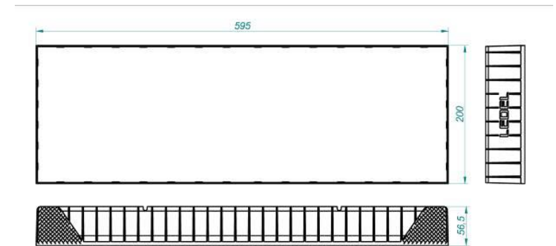
Рисунок 1а Светильники «L-school 16»
