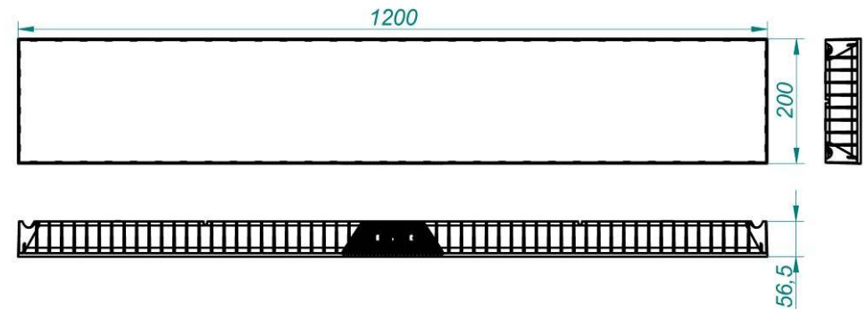
Рисунок 1б Светильник «L-school 32»
