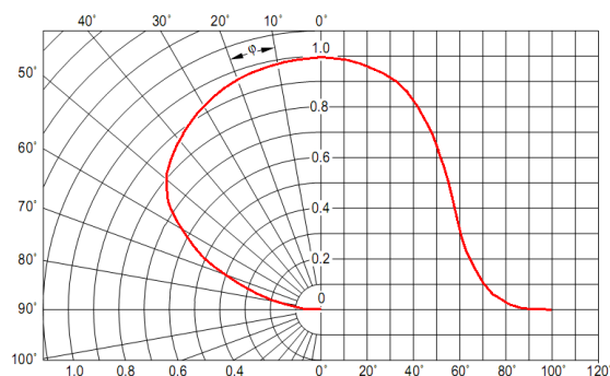
Рисунок 3 Тип КСС в исполнении «Д»
