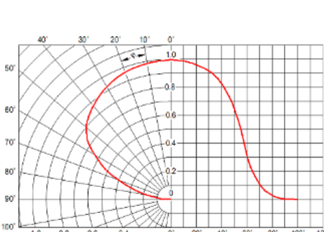
Рисунок 4 Типы КСС
