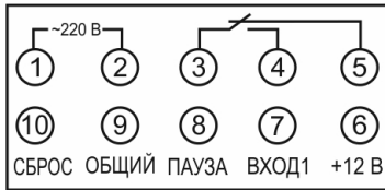
Рис. 6 Схема подключения ARCOM-TC-D44
