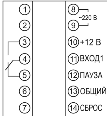
Рис. 7 Схема подключения ARCOM-TC-D77
