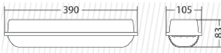
Рисунок 1. Внешний вид
