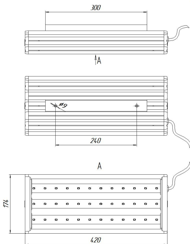
Светильник УСС 48 с 2Ех маркировкой потолочное крепление
