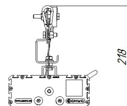
Светильник УСС 60 МАГИСТРАЛЬ Ш с 2Ех маркировкой крепление на трос
