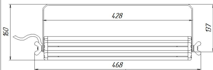
Светильник УСС 60 МАГИСТРАЛЬ Ш с 2Ех маркировкой крепление скоба
