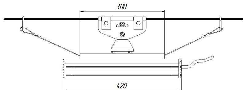
Светильник УСС 60 МАГИСТРАЛЬ Ш с 2Ех маркировкой крепление на трос
