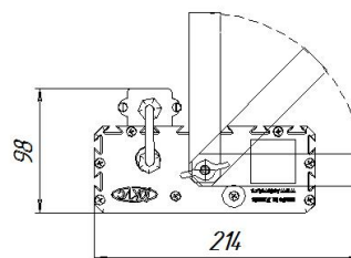
Светильник УСС 90 МАГИСТРАЛЬ Ш с креплением скоба
