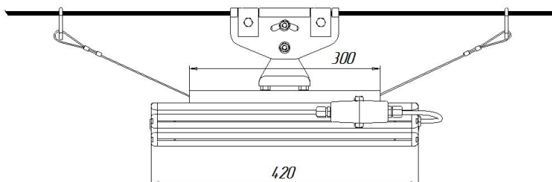
Светильник УСС 90 МАГИСТРАЛЬ Ш крепление на трос
