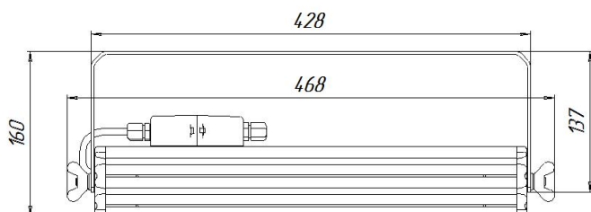
Светильник УСС 90 МАГИСТРАЛЬ Ш с креплением скоба
