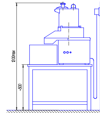
Рисунок 14 - Установка машины
