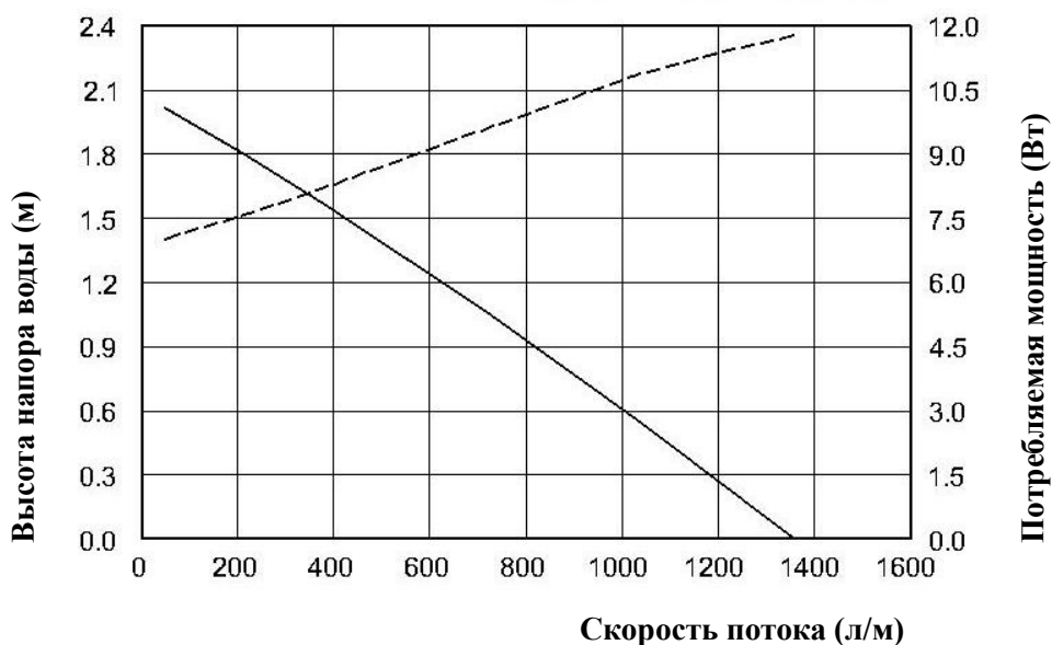
График работы насоса
