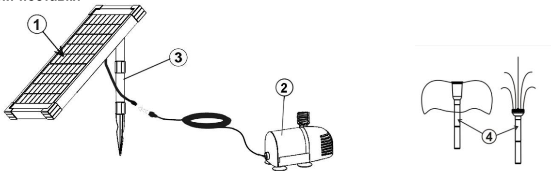
1) Солнечная батарея 2) Насос, работающий от солнечной энергии 3) Шип 4) Насадки
