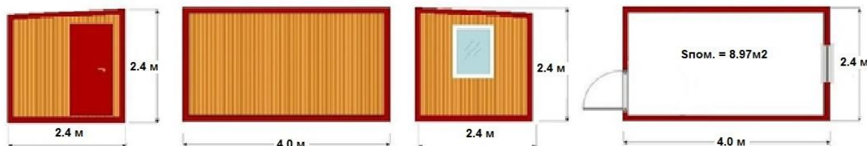
БС-03-4.0 (торцевой вход и окно, без тамбура)
