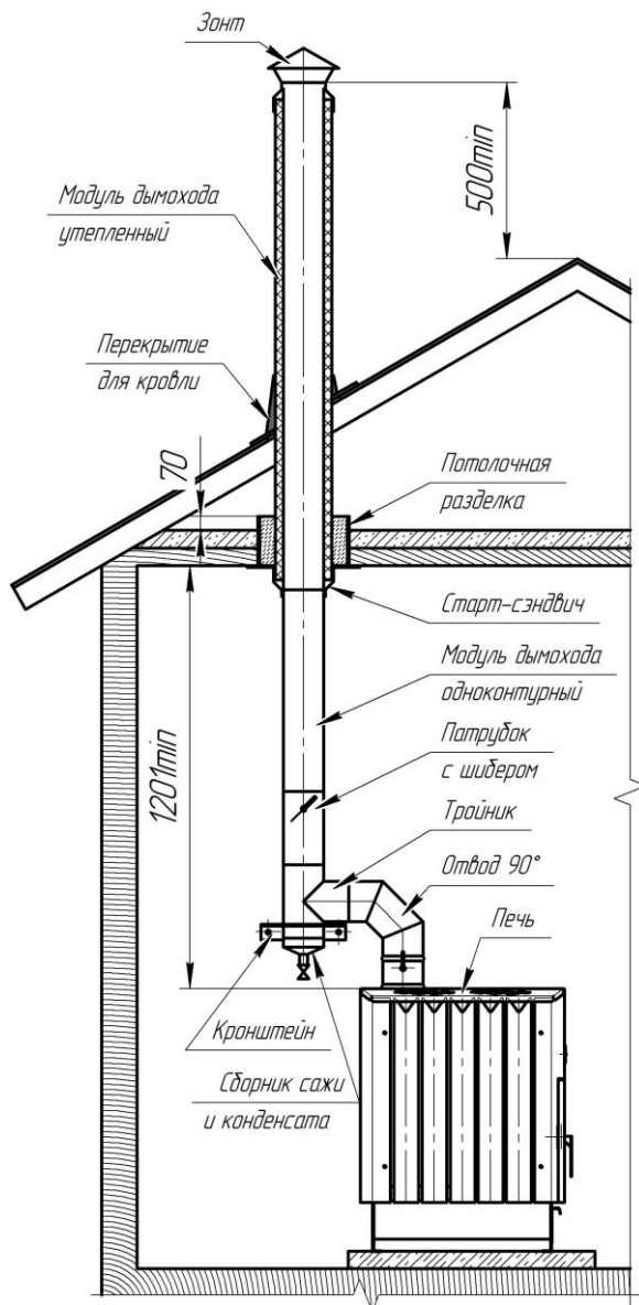
Установка печи
