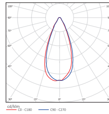
Угол излучения 60°
