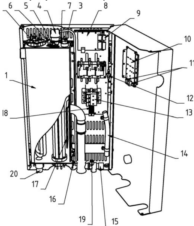
Рис. 4 Устройство прибора
