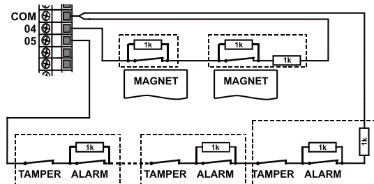
Рисунок: Пример подключения других детекторов к одному входному терминалу при двойной балансировке шлейфа резистором 1k. Подключение 2 магнитных контактов к входным терминалам 4-COM. Подключение детекторов с тревожными и тамперными контактами к входным терминалам 5-COM.
