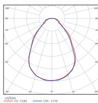
Рассеиватель «Призма»
