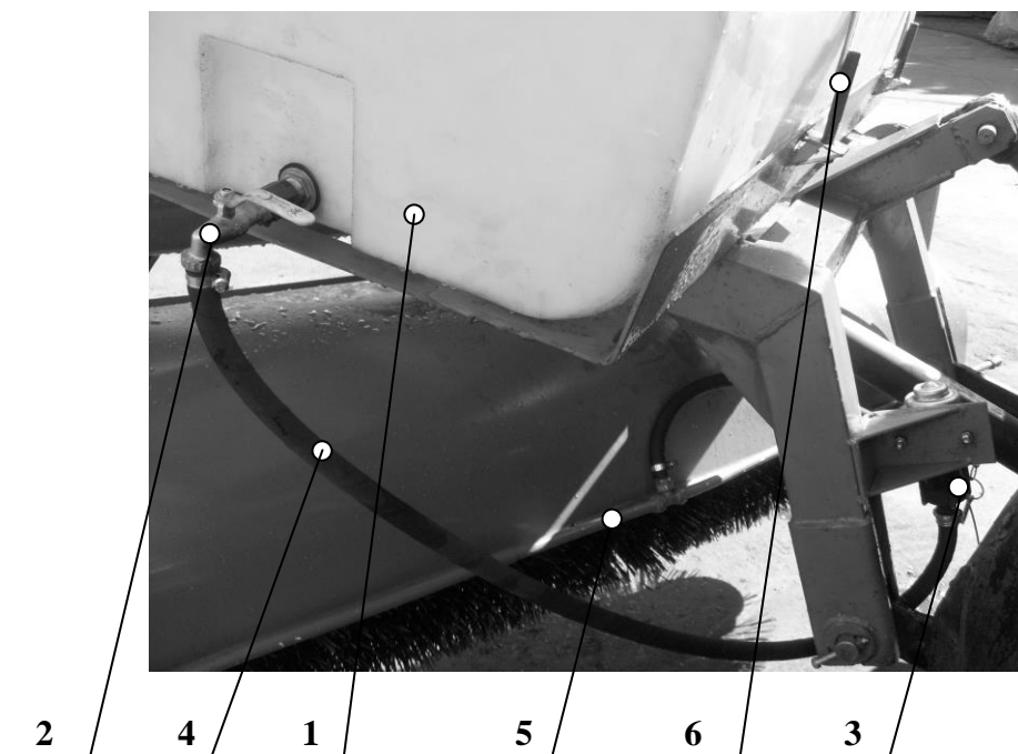
Рисунок 3. Основные узлы гидросистемы орошения Оборудования щеточного исполнения УМДУ- 80/82.02 ГО
