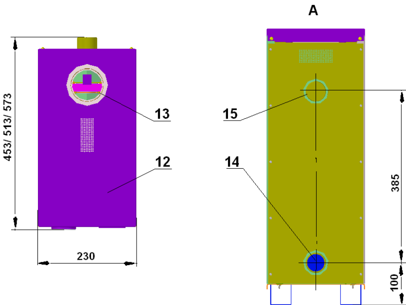
Рис.1 Котлы КС-Г-7S-Э/10S-Э/12S-Э
