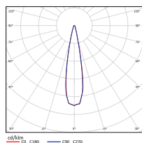
Угол излучения 10°
